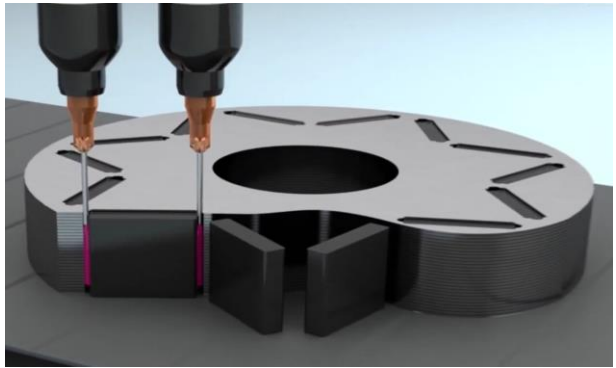
Epoxy 흐름성 조정으로 바닥면 Plate 불필요
